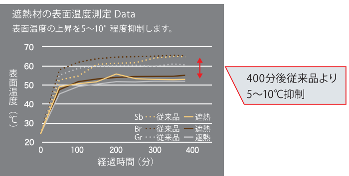
[ 遮熱材の表面温度測定DATA ]
