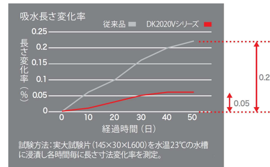
デッキ浸水過酷試験結果
